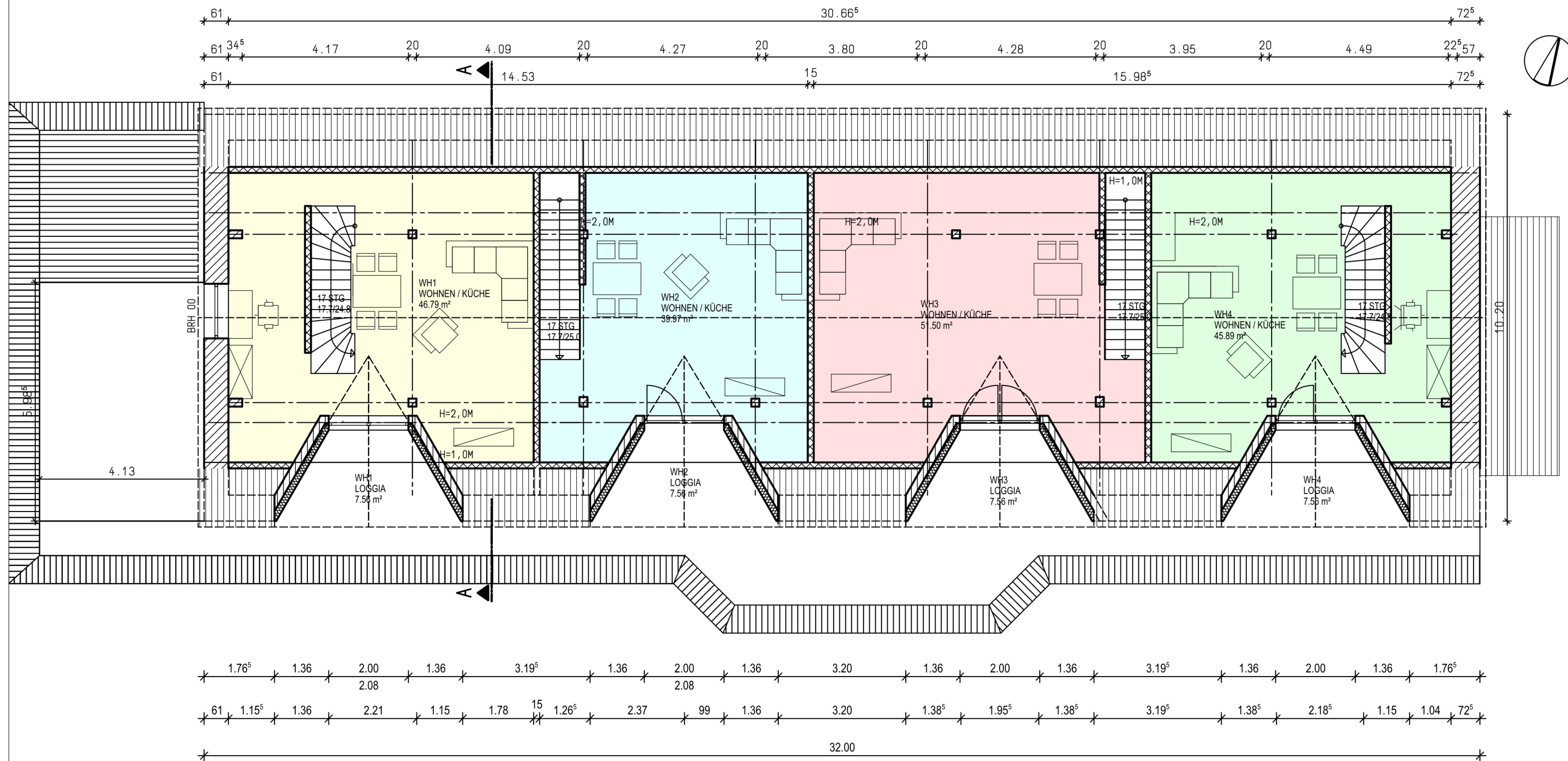
GRUNDRISS DACHGESCHOSS
