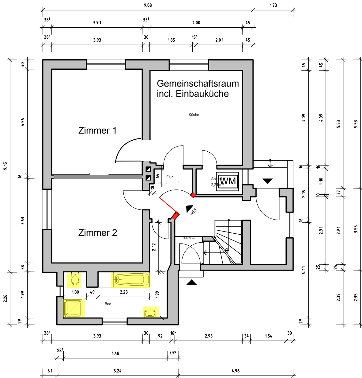
Grundriss Erdgeschoss, M 1 : 100
