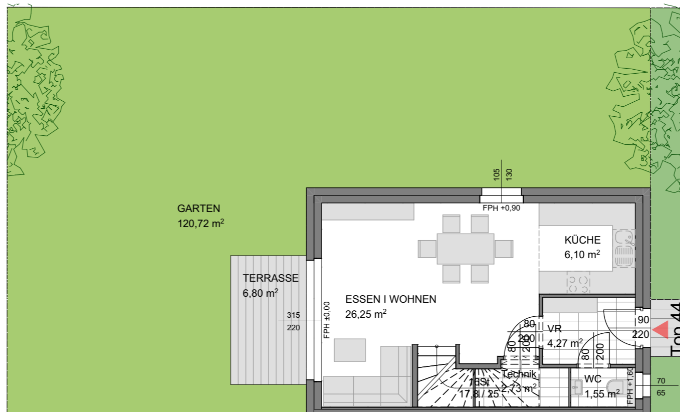
Erdgeschoss
