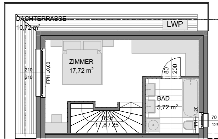
Dachgeschoss
