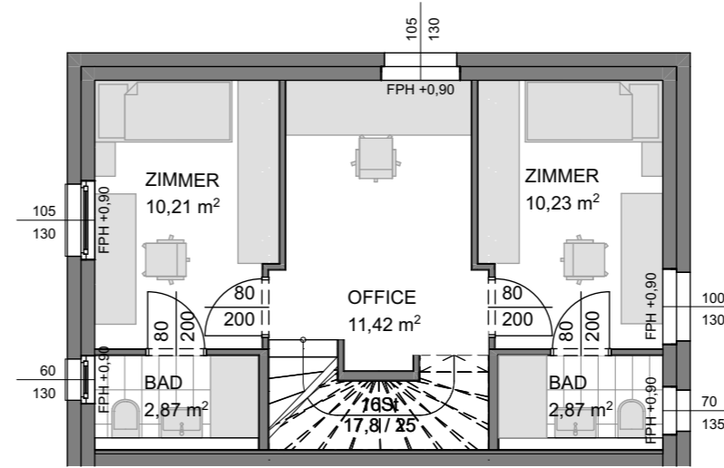
Obergeschoss
