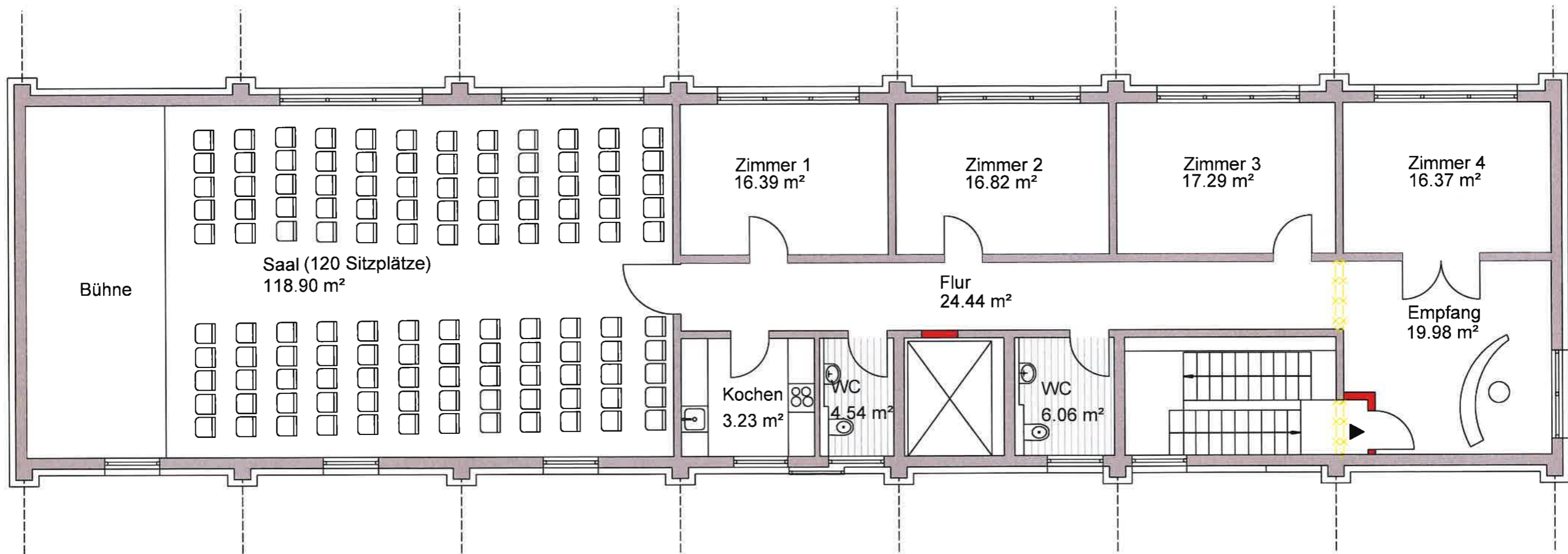
Grundriss Obergeschoss
