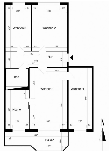
Grundriss mit Balkon
