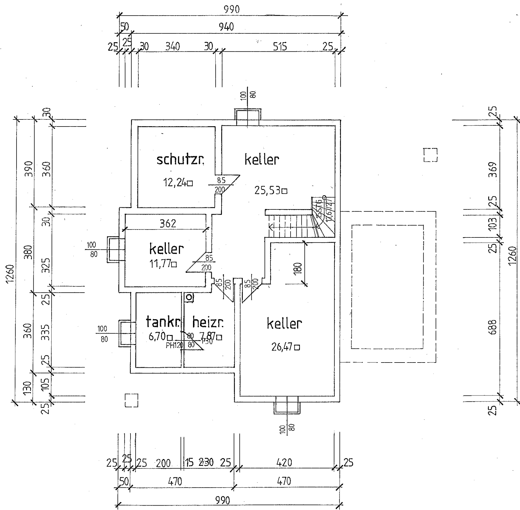
KELLERGESCHOSS 90,58m 2
