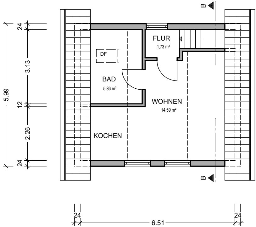
_dachgeschoss_
