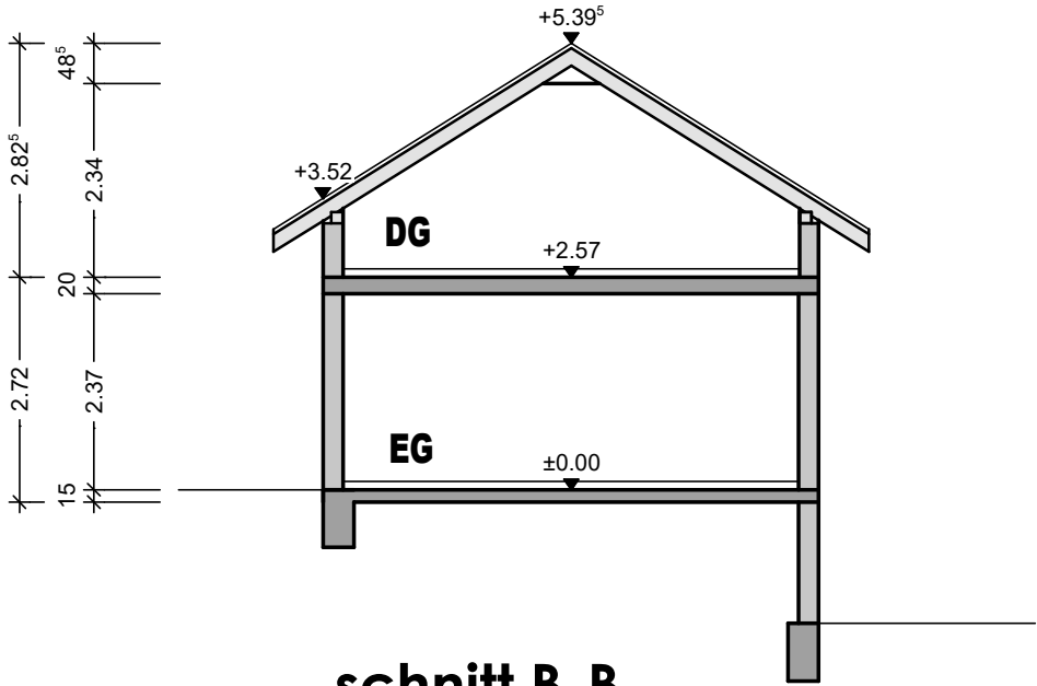
_schnitt B-B_
