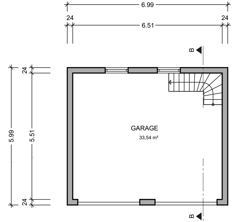
_erdgeschoss_
