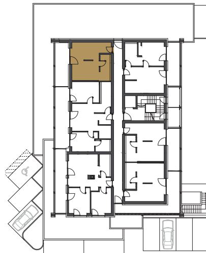
Plan 1. Obergeschoss
