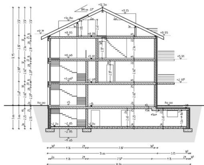
SCHNITT b-b M1:100
