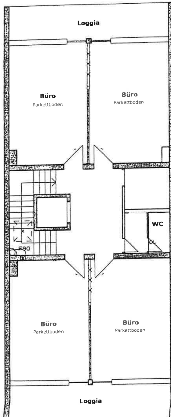
Grundrisszeichnung 5. Obergeschoss (kein Maßstab)
