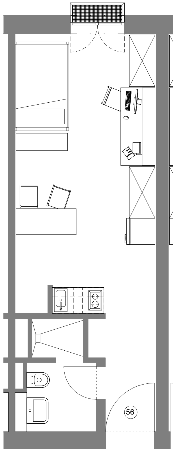
WE 56 - 2. Obergeschoss
