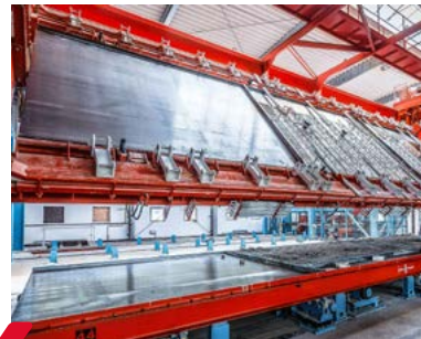
6 Einwenden der Wandschalen
