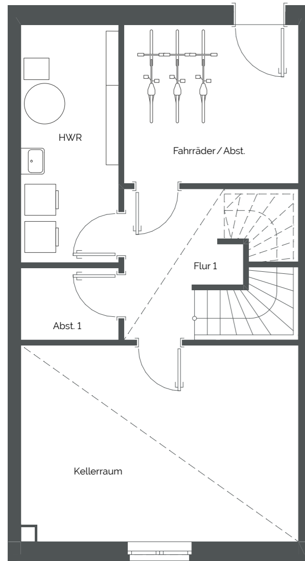
Kellergeschoss
