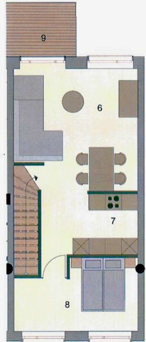
1. Obergeschoss
