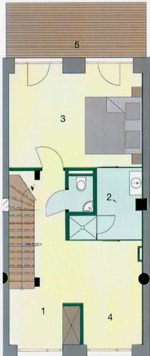
Eingang Erdgeschoss
