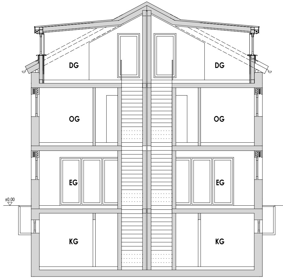
Schnitt A - A
