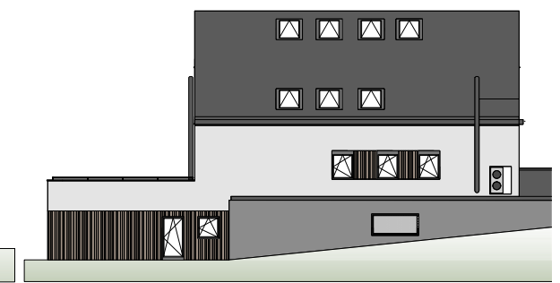
Ansicht Süd
