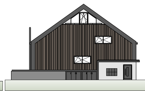
Ansicht Ost
