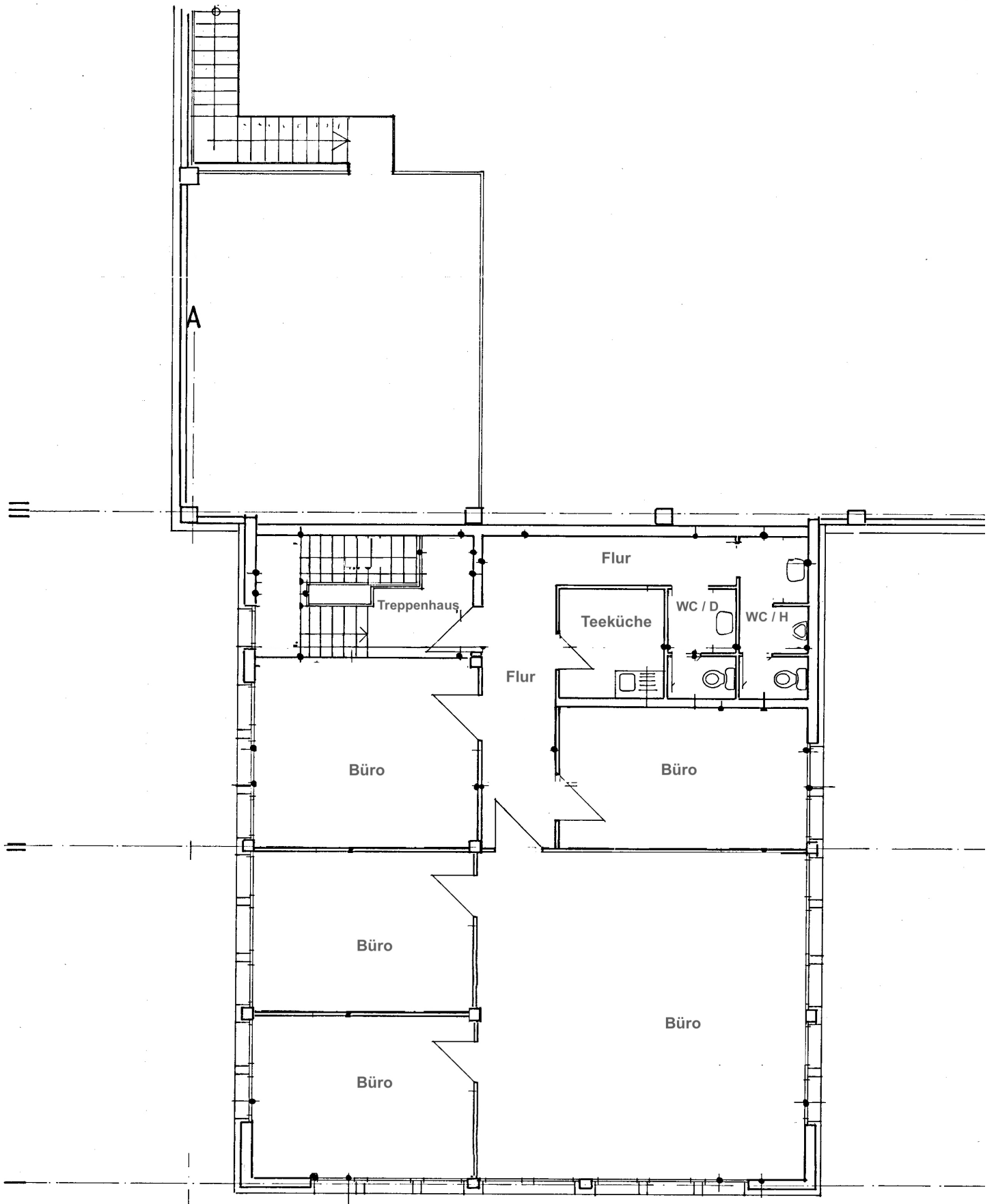
Büroflächen Gebäude 9 A, Obergeschoss Nutzflächen ca. 168 m 2
