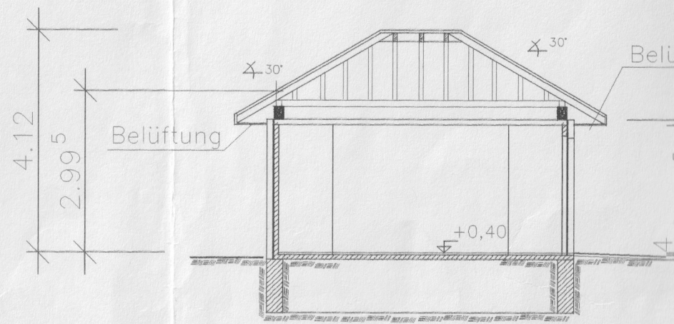
Schnitt A-A
