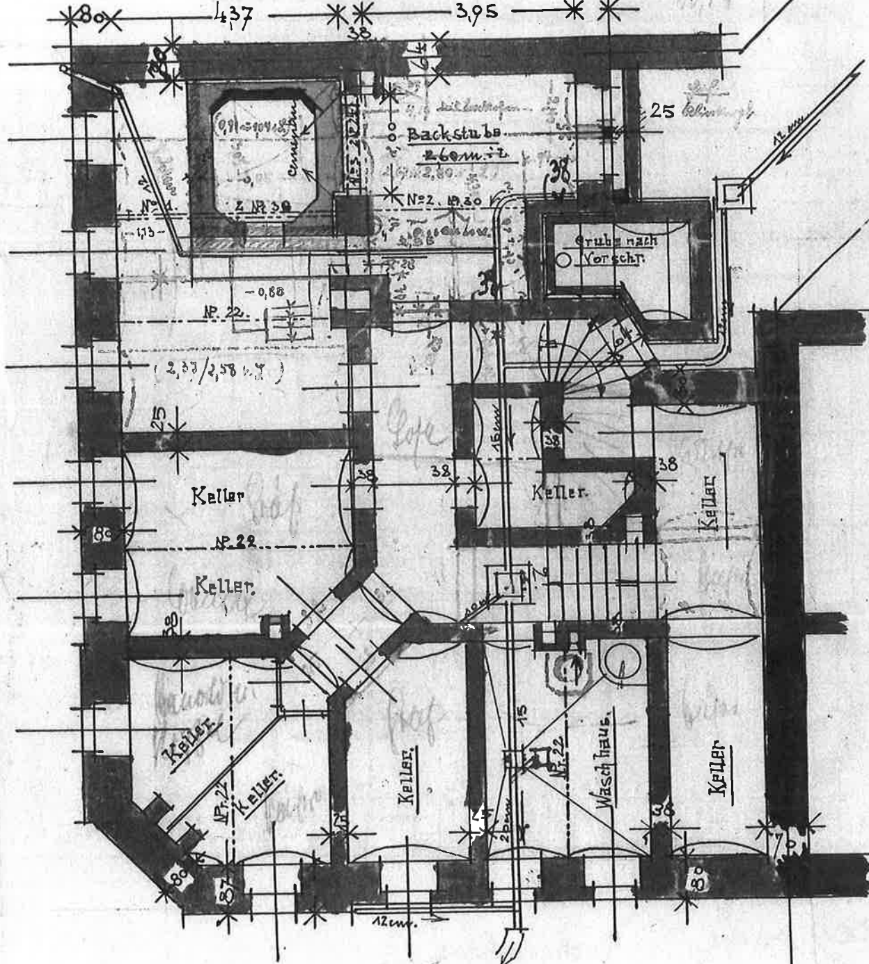
Kellergeschoss.
