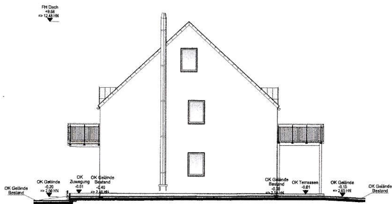
Ansicht West M 1 : 100
