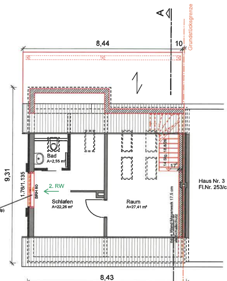
GRUNDRISS DACHGESCHOSS
