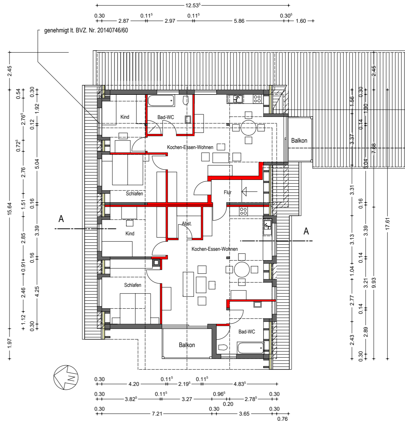
Dachgeschossgrundriss
