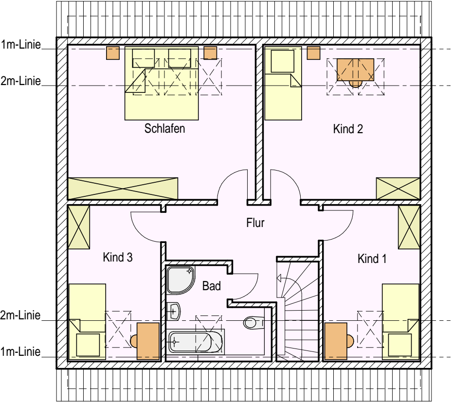
Typengrundriss
