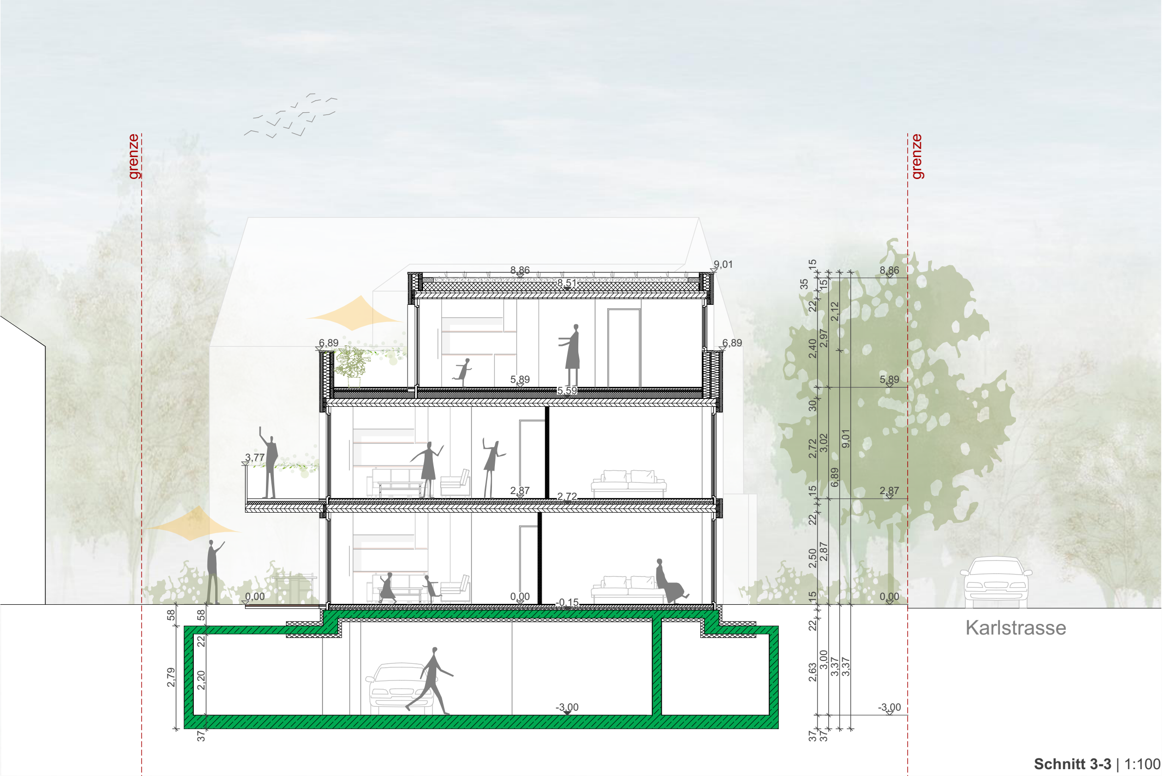
Schnitt 3-3 | 1:100
