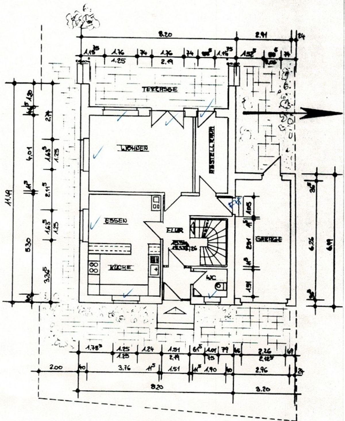
ERDGESCHOSS M. 1:100
