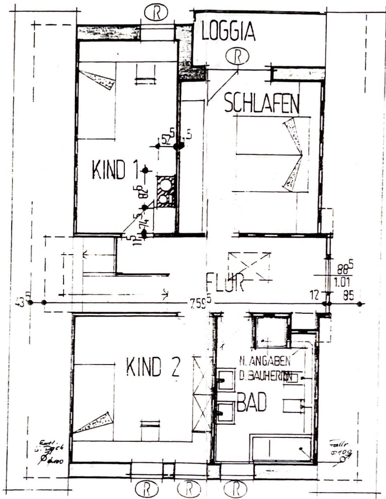
AUSBAU : 2. BAUABSCHNITT
