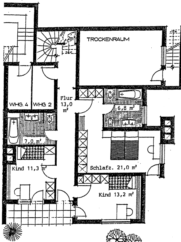
Wohnung 2: UNTERE EBENE 73,5 qm
