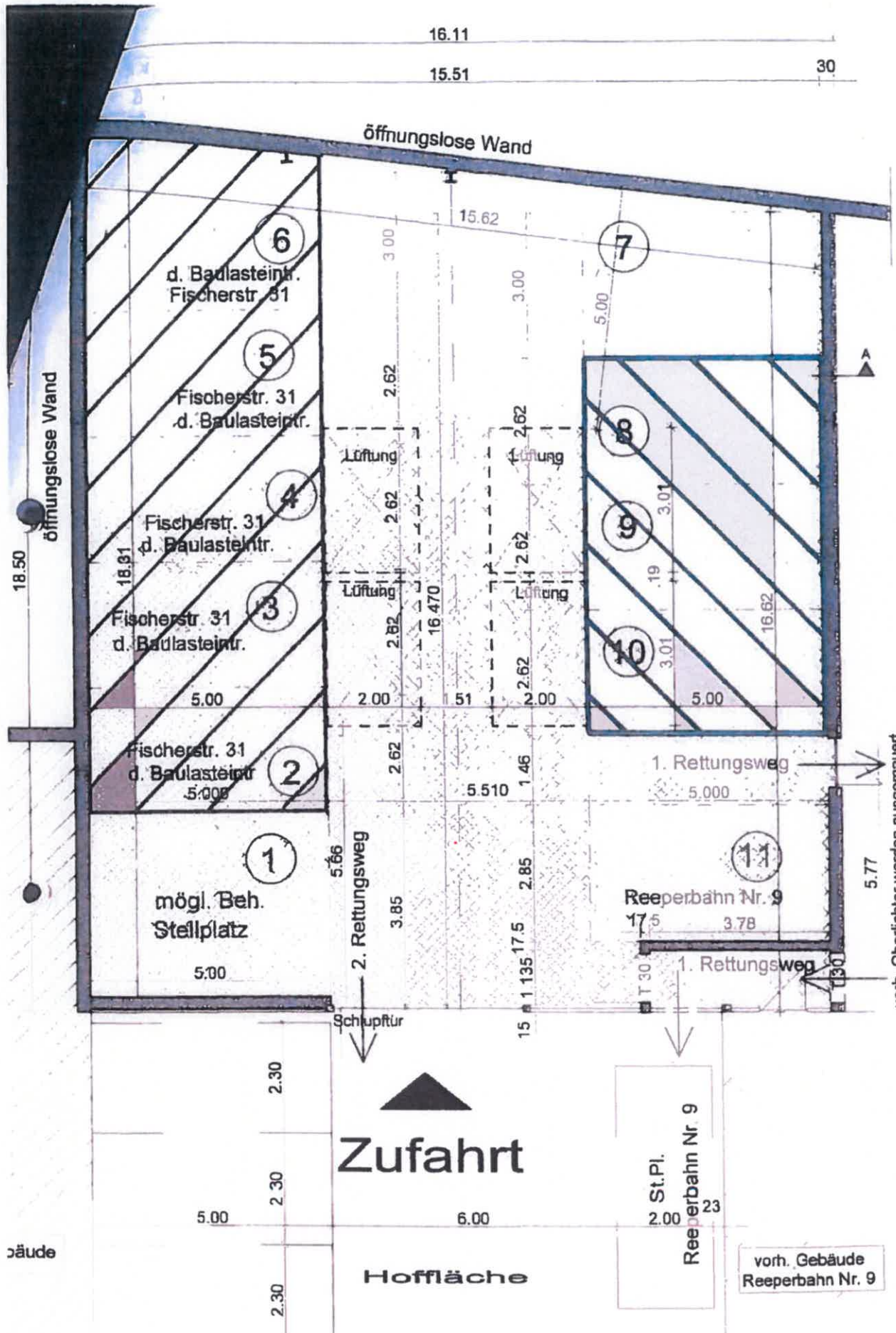
Grundriss
