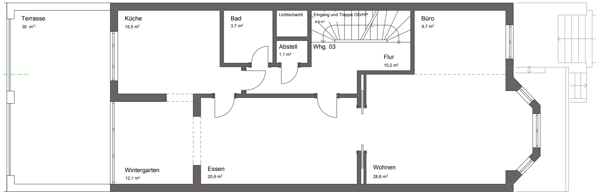
Grundriss 1. Obergeschoss
