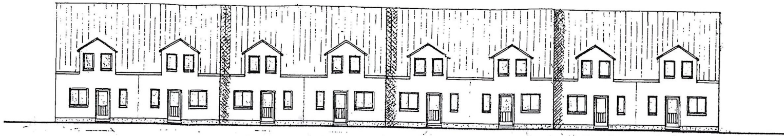
Straßenansicht (Am neuen Friedhof) M. 1:200
