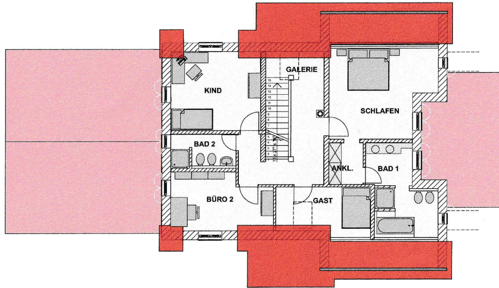
DACHGESCHOSS M 1:100
