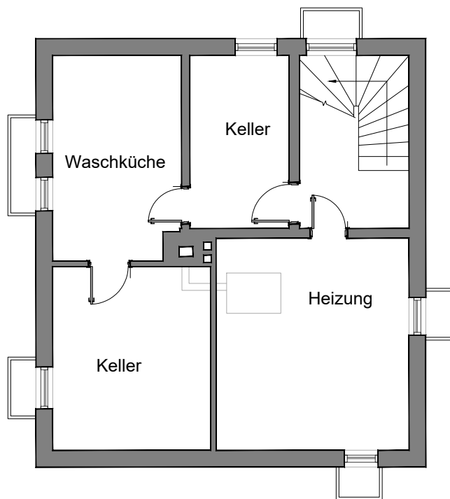
Kellergeschoss
