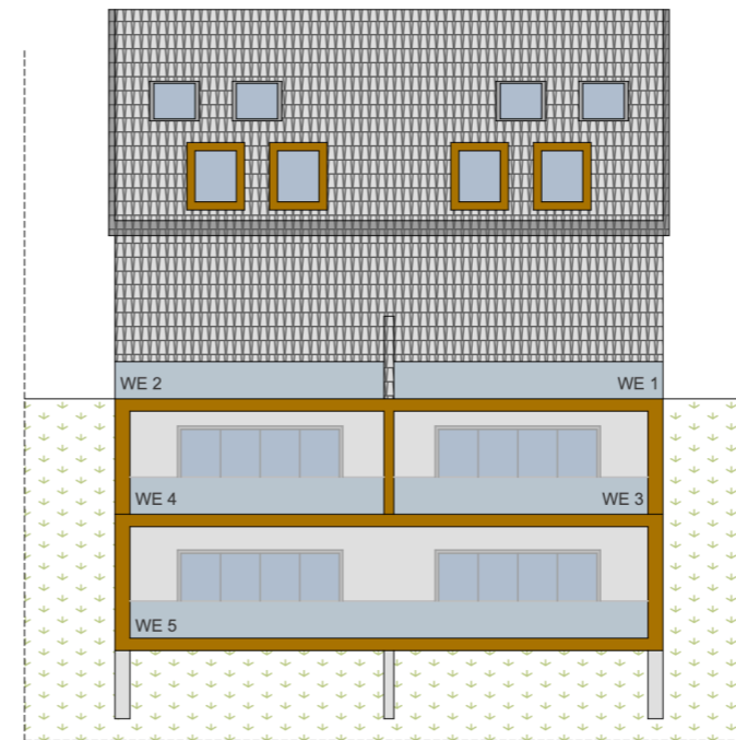
Ansicht Süd-West
