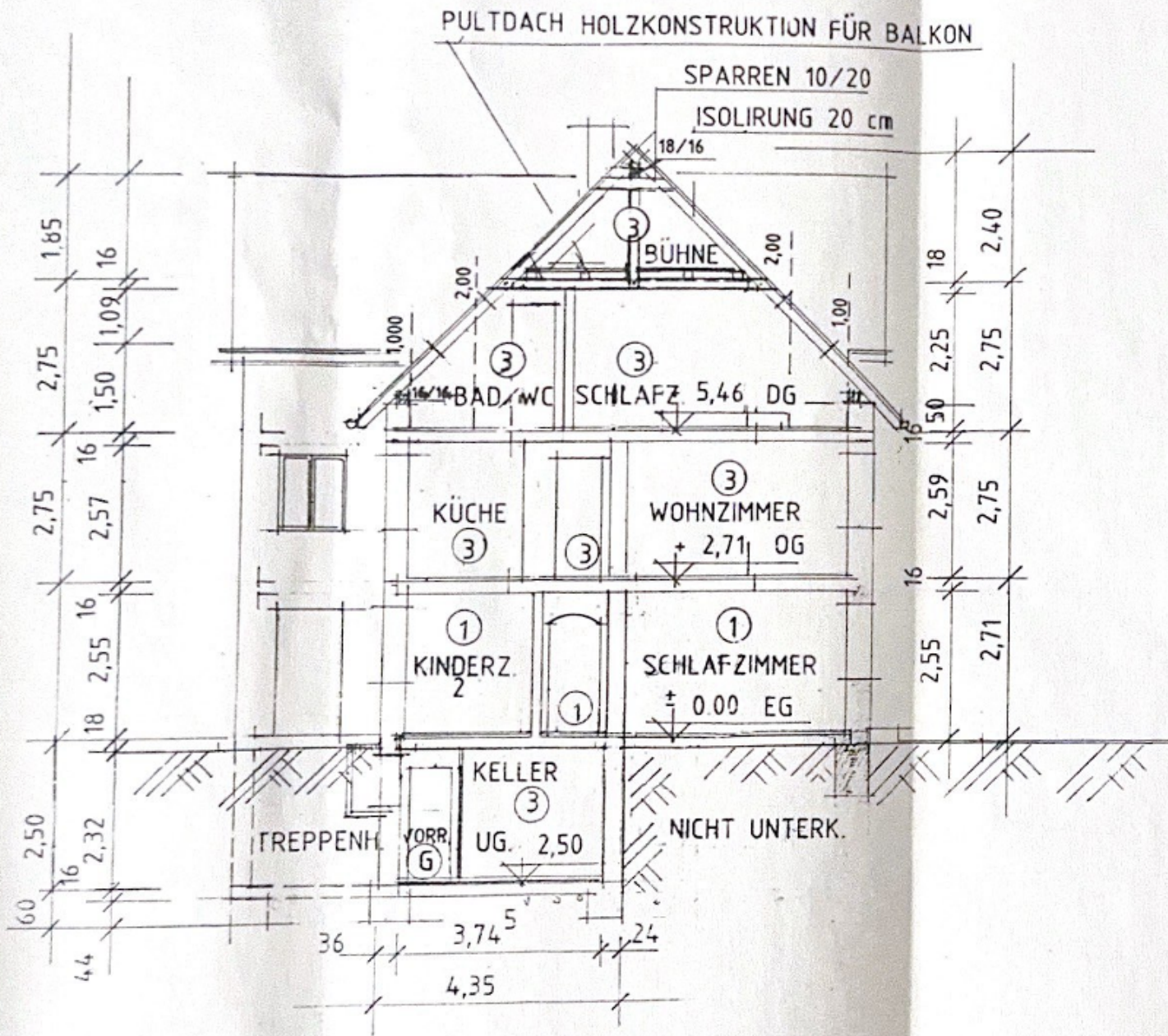
SCHNITT A-B
