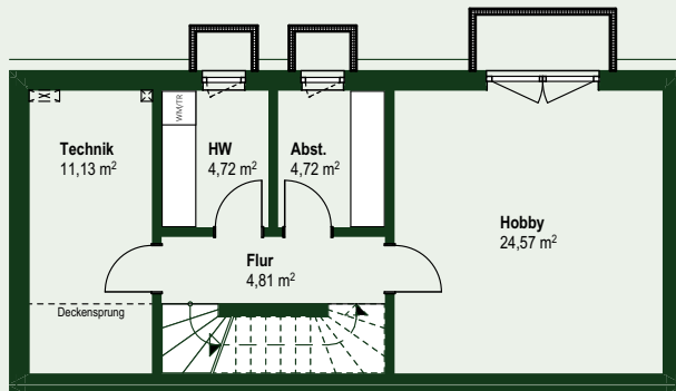
KELLERGESCHOSS
