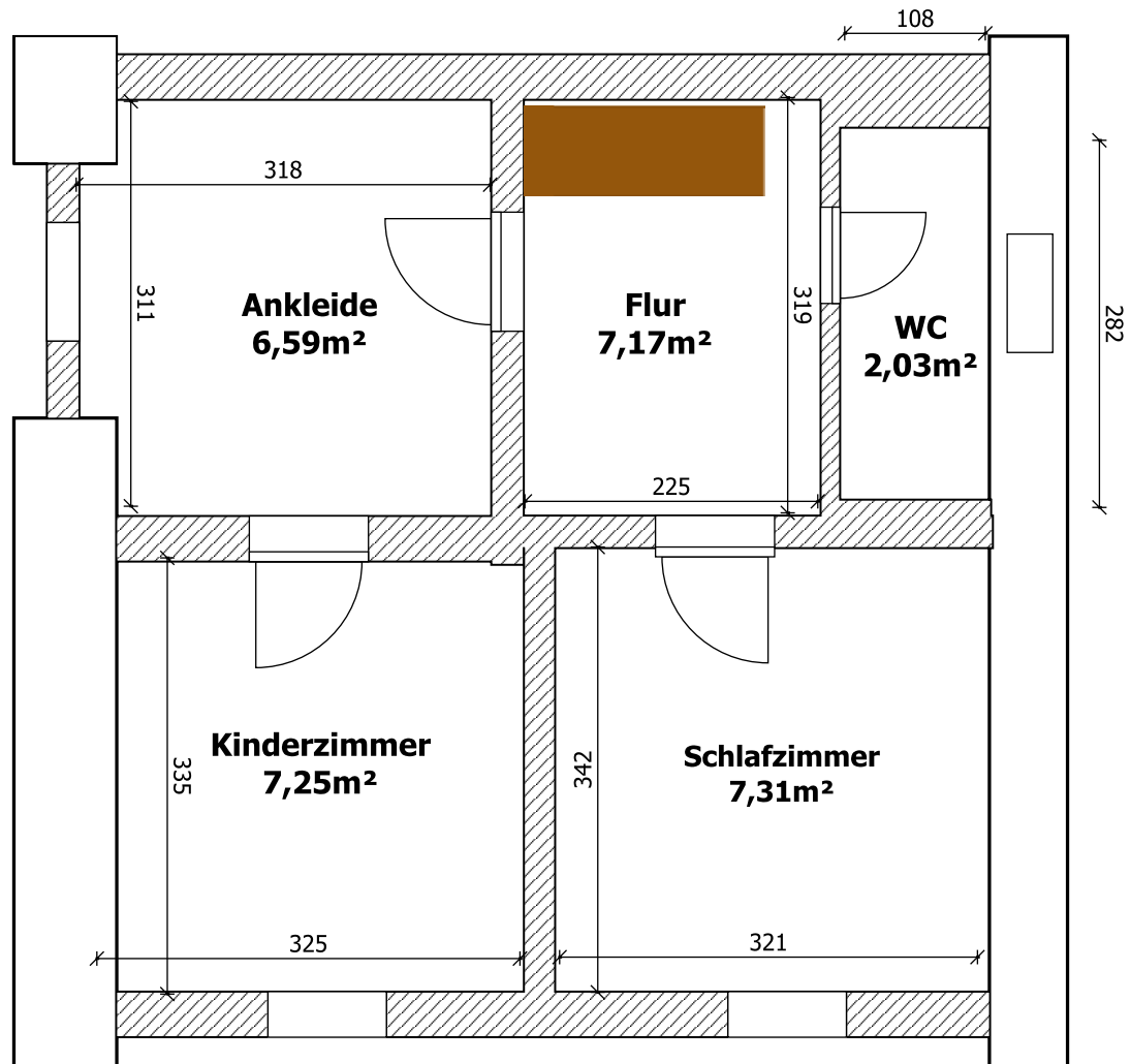
Zeit, Am Wiesengrund 14 Grundriss Dachgeschoß Raumhöhe 2,20m, Drenpelhöhe 1,20m
