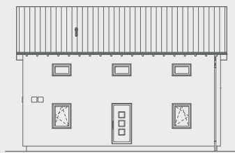
Ansicht Eingang
