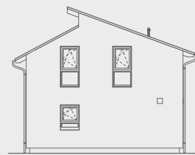
Ansicht Links
