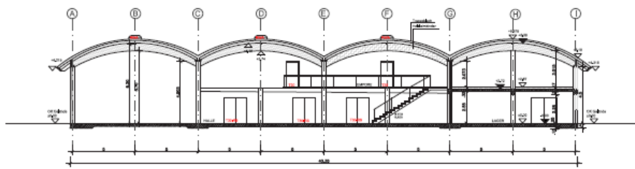
SCHNITT A - A
