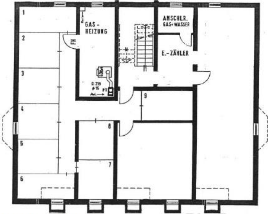
Grundriss Kellergeschoss
