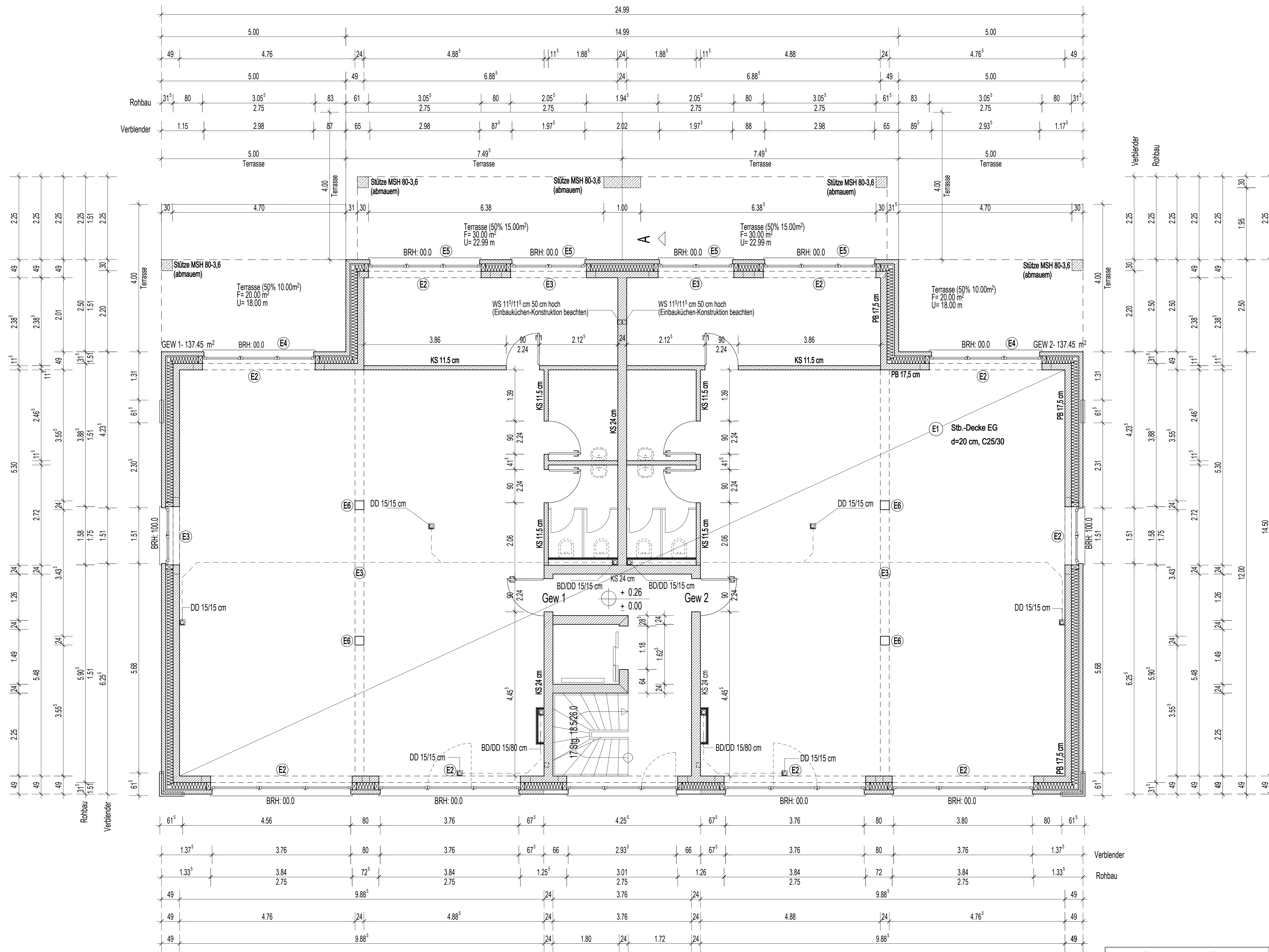
Erdgeschoss-Grundriss
