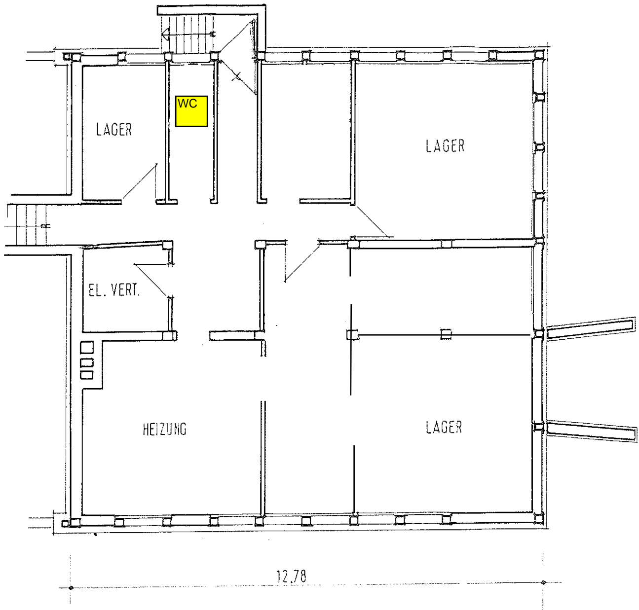
GRUNDRISS - KELLERGESCHOSS
