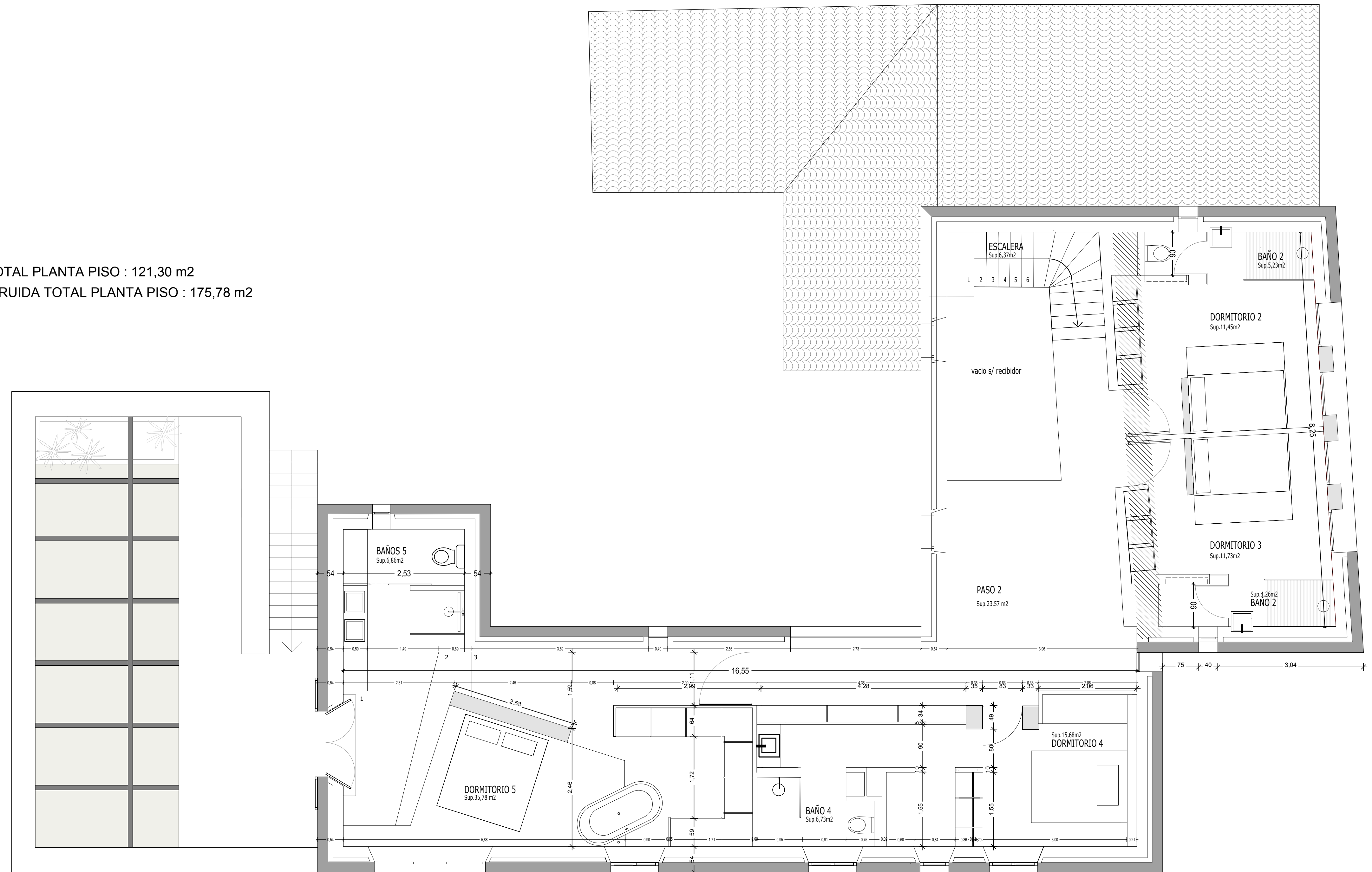
PLANTA PISO
