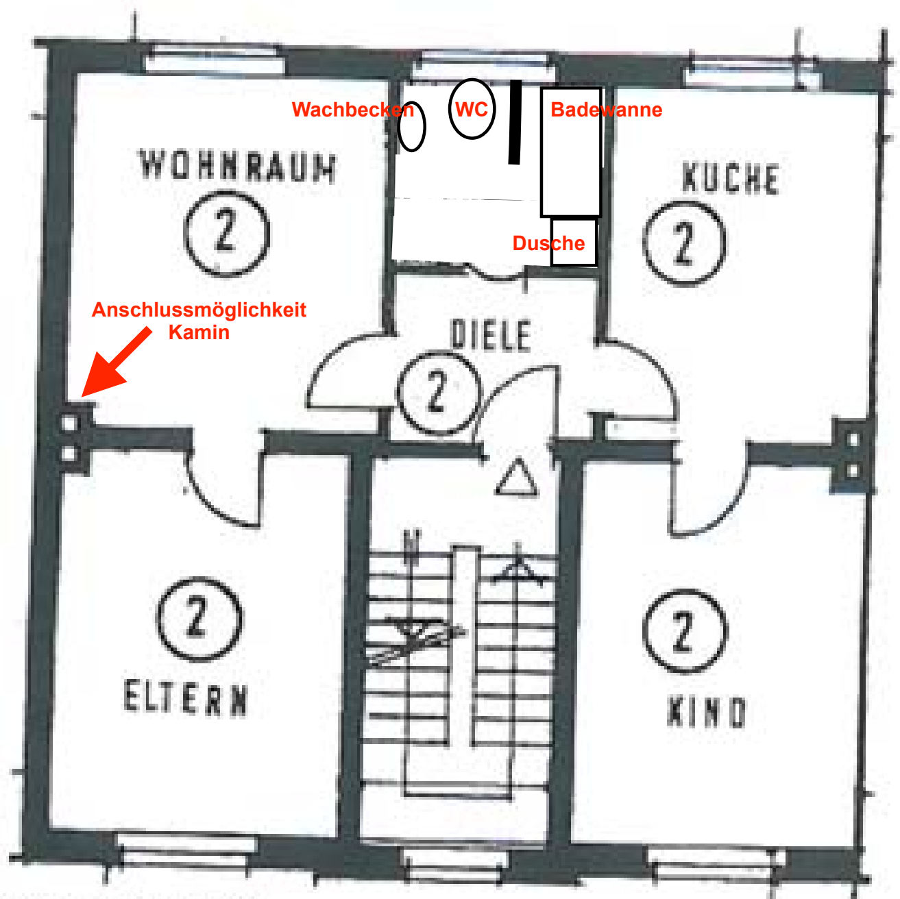
Grundriss 1. OG
