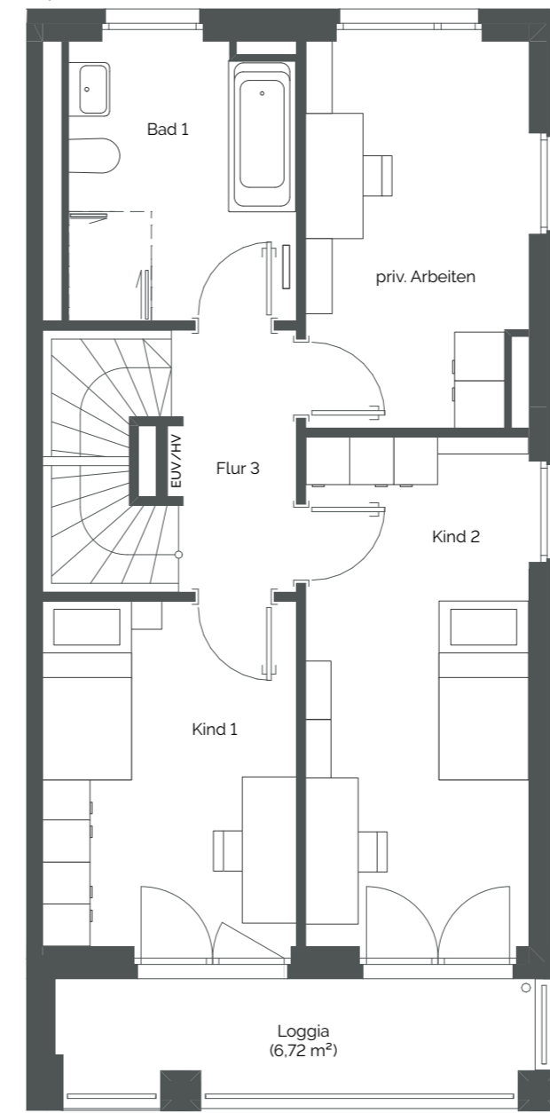
1. Obergeschoss
