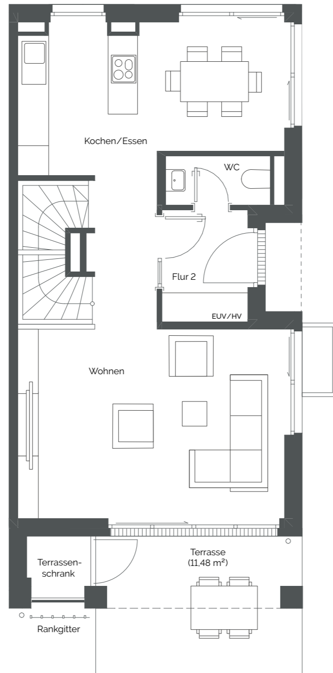
Erdgeschoss
