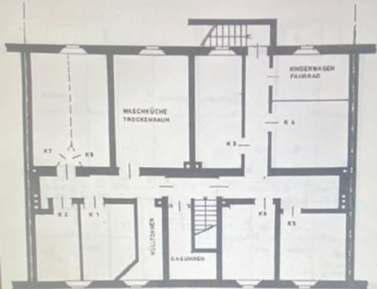
KELLERGEOSCHOSS M 1:100
