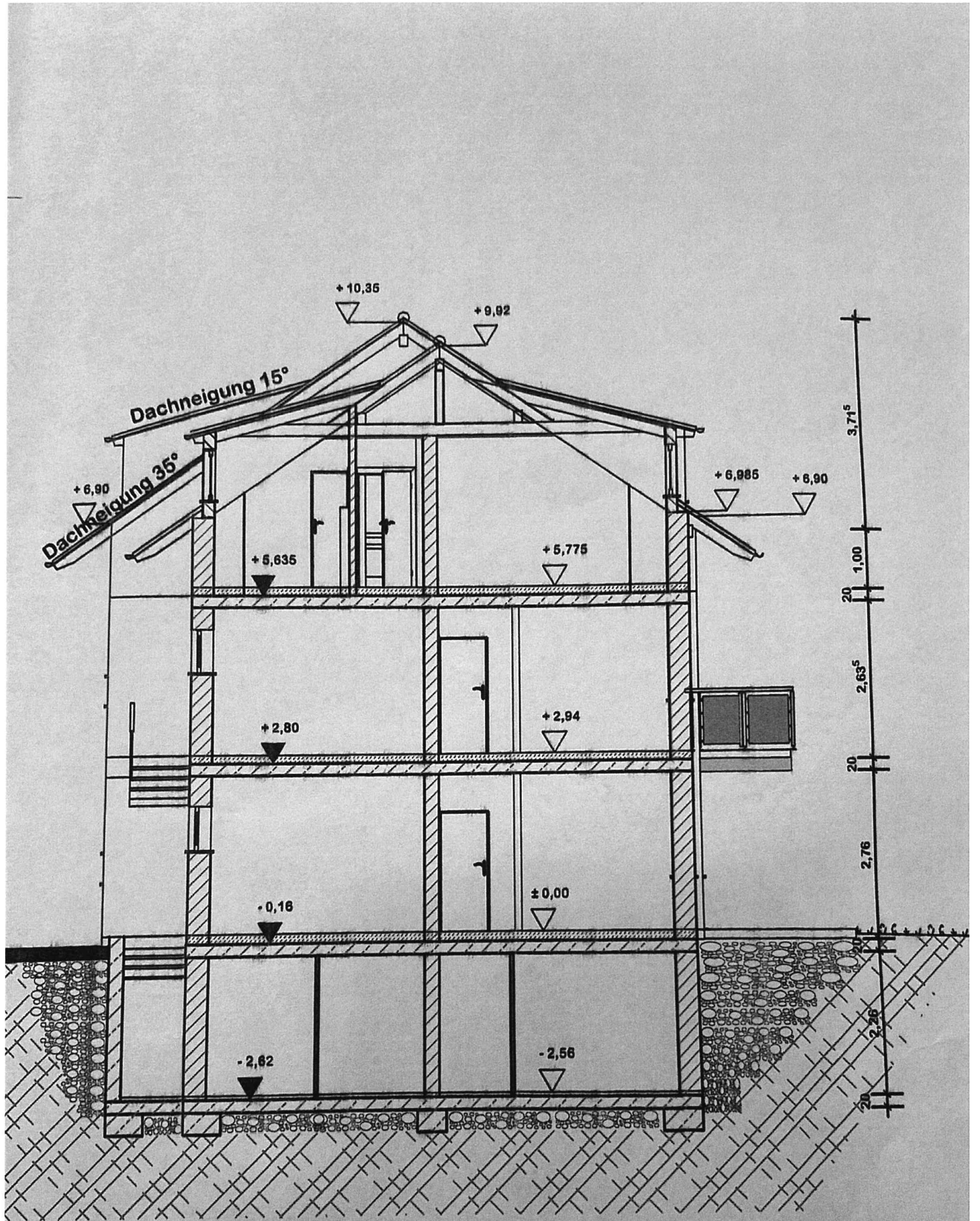
Schnitt A - A
