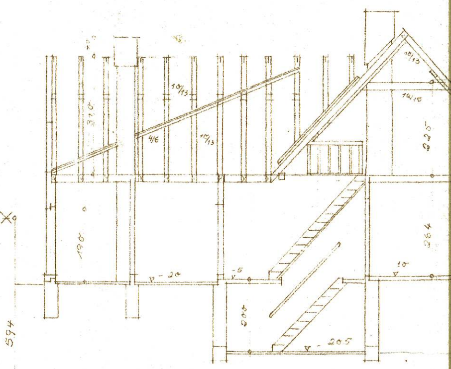
Dachstuhl
