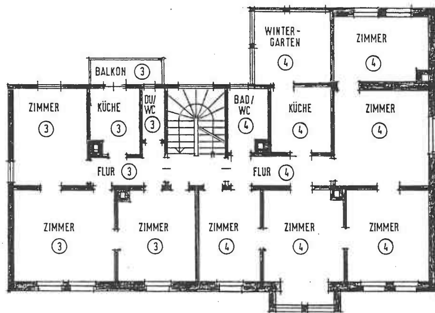
1. OBERGESCHOSS M. 1/100
