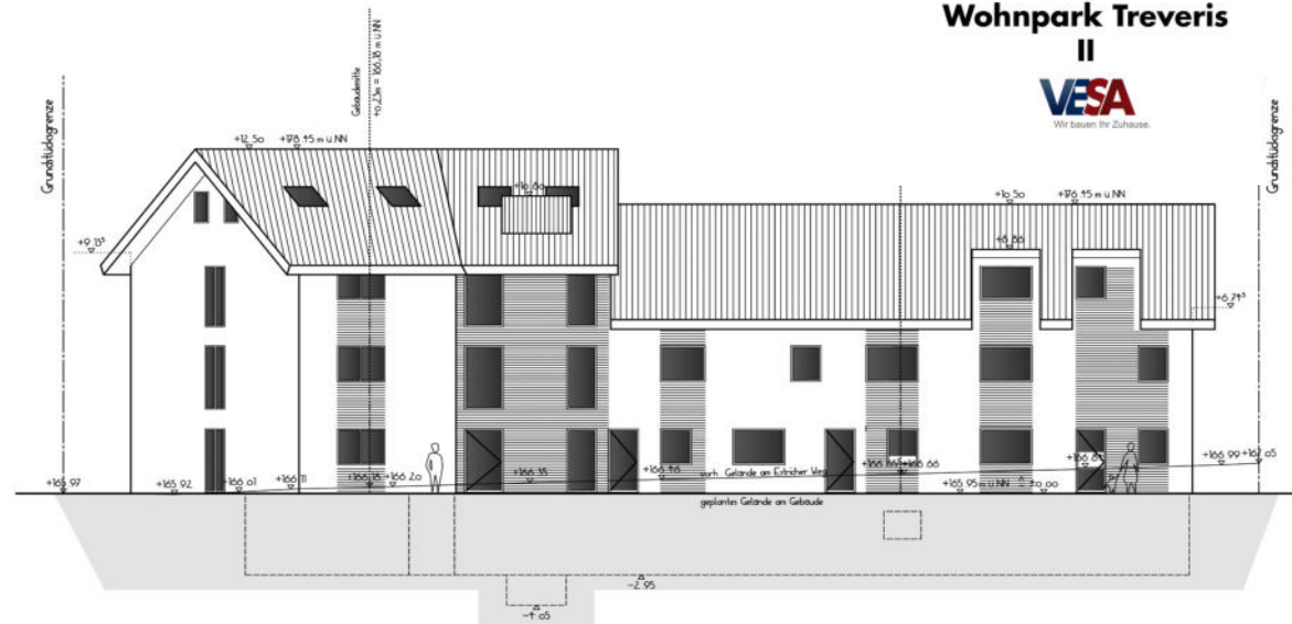
HAUS 1 - ANSICHT ESTRICHERWEG - ANSICHT NORD-WEST M 1:100
