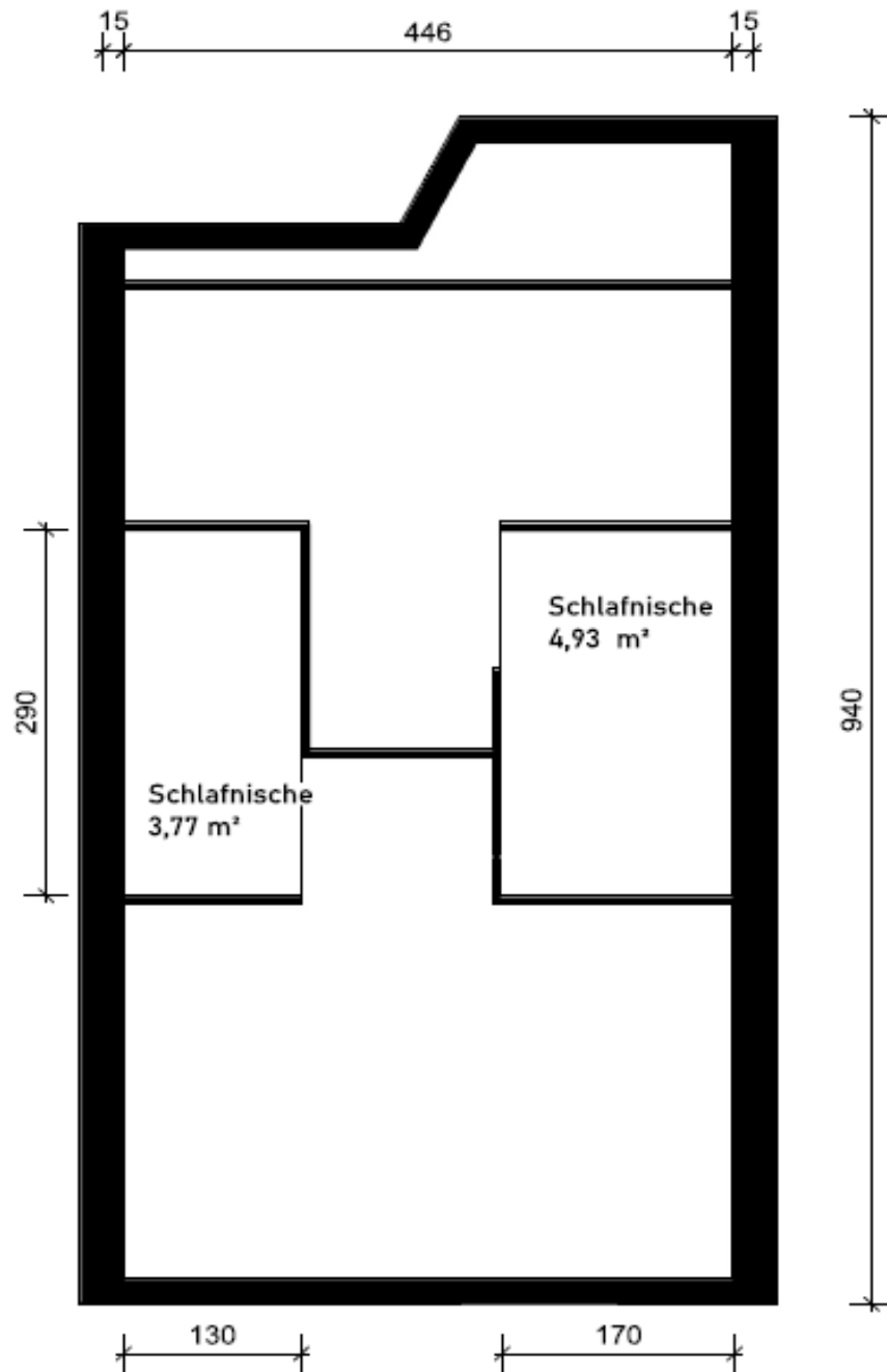
Grundriss Spitzboden
